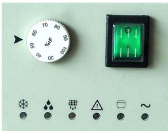
Панель управления
