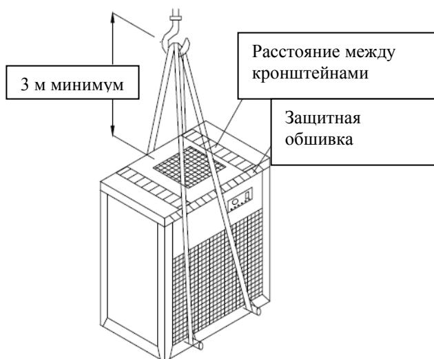
Подъем краном
